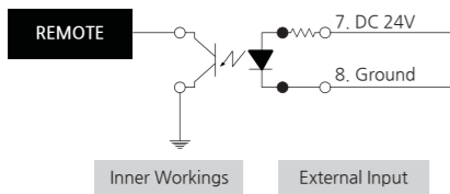
Circuit(DC 24V Input)
